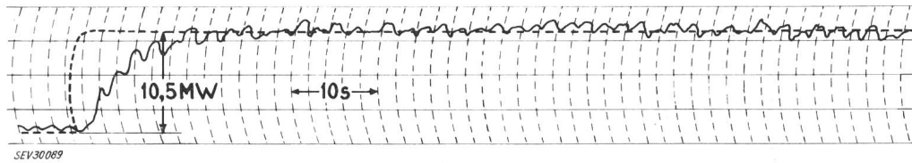
Fig. 4 Groupe de 85 MW de la Centrale de Chastang d'EdF
