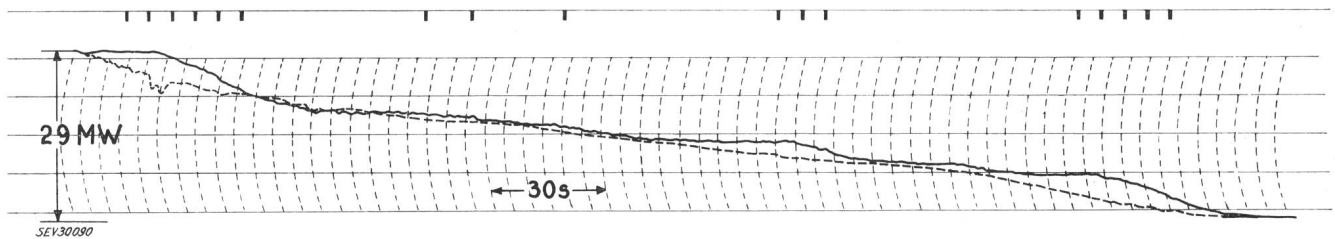
Fig. 5 Groupe de 85 MW de la Centrale de Chastang d'EdF
