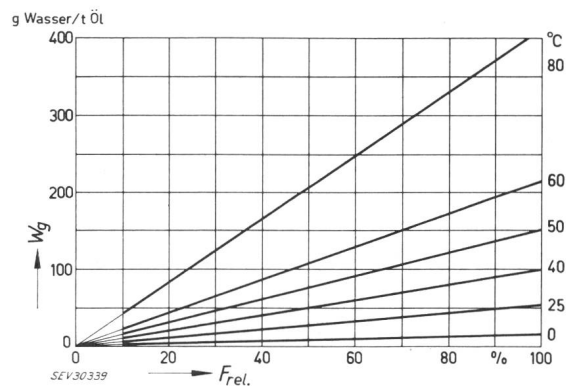
Fig. 2 Wassergehalt W_g des Öles in Abhängigkeit von der relativen Feuchtigkeit F_{rel} . Parameter ist die Öltemperatur
