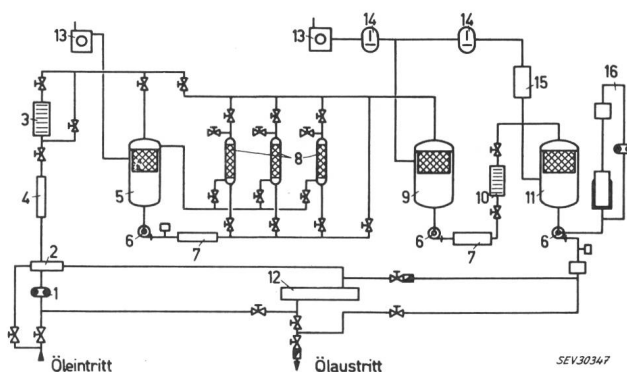
Fig. 10 Kombinierte Aufbereitungs- und Regenerier-Anlage 1 Förderpumpe; 2 Mengenregler; 3 Filterpresse; 4 Kühler; 5 Entgasungskessel 1. Stufe; 6 Umwälzpumpen; 7 Ölwärmer 25 kW; 8 Fullerkessel; 9 Entgasungskessel 2. Stufe; 10 Filterpresse; 11 Entgasungskessel 3. Stufe; 12 Ölwärmer 120 kW; 13 Drehschieberpumpen S = 100 \text{ m}^3/\text{h} ; 14 Rootspumpen S = 1600 \text{ m}^3/\text{h} ; 15 Kondensator; 16 Inhibieranlage
