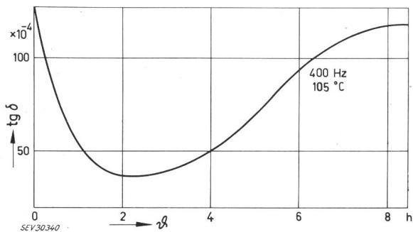
Fig. 3 Zeitverlauf einer Verlustfaktor-Messung \phi Zeit
