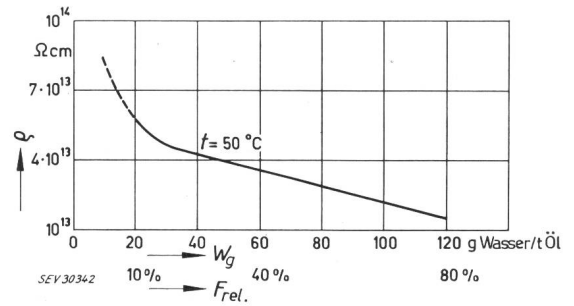
Fig. 5 Abhängigkeit des spezifischen Widerstandes \rho vom Wassergehalt W_g des Öles Die Kurve gilt für ein gebräuchliches Transformatoröl
