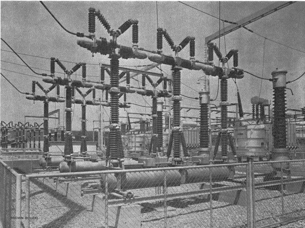
Teil der 220-kV-Freiluftanlage Laufenburg/Schweiz mit 220-kV-Druckluftschneellschaltern. Im Hintergrund eine einphasige Auto-Stufentransformatorgruppe für 125 MVA, 220/150kV.
