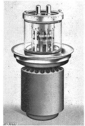
Fig. 5 Senderöhre mit Verdampfungskühlung
