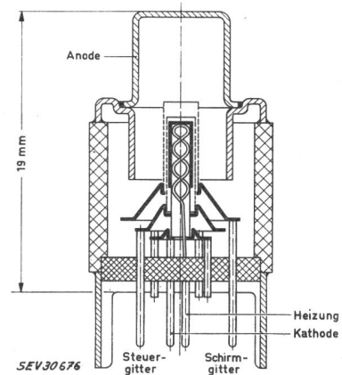
Fig. 16 Nuvistor-Kleinsignal-Tetrode
