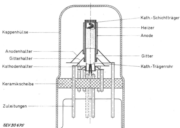
Fig. 15 Nuvistor
