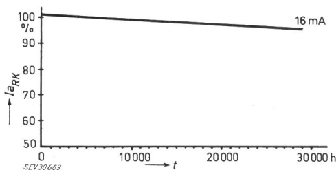
Fig. 9 Lebensdauermessungen an C3m-Röhren I_{aRK} Anodenstrom; t Zeit
