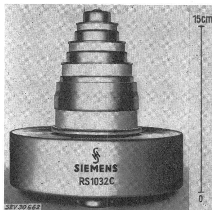
Fig. 2 Luftgekühlte Sendetetrode für Fernsehsender Keramikausführung
