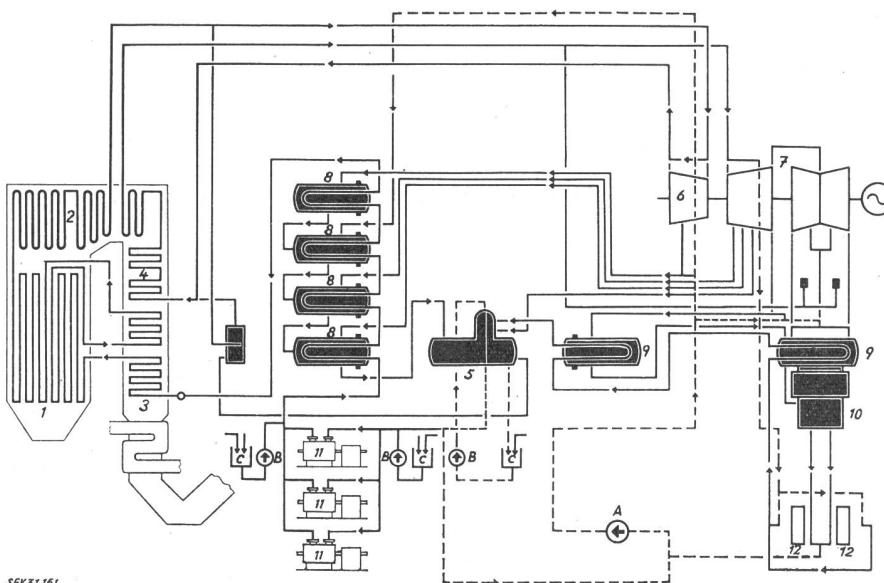
Fig. 2 Beizkreisläufe einer thermischen Anlage mit Zwangsdurchlaufkessel 1 Brennkammer; 2 Überhitzer, hängend; 3 Economiser; 4 Zwischenüberhitzer; 5 Speiswasserbehälter; 6 Hochdruck-Turbine; 7 Niederdruck-Turbine; 8 Hochdruck-Vorwärmer; 9 Niederdruck-Vorwärmer; 10 Kondensator; 11 Hochdruck-Kesselspeisepumpe; 12 Kondensatpumpe; A Borg-Zirkulationspumpe; B Borg-Chemikalien-Dosierpumpe; C Chemikalien-Mischtank 1...4 Zwangsdurchlaufkessel
