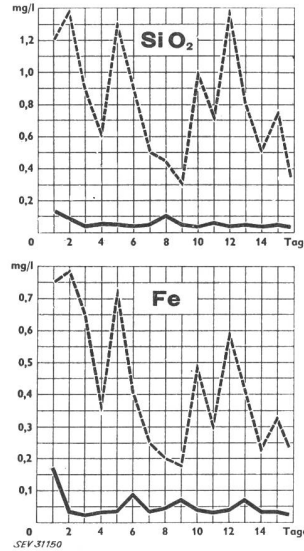
Fig. 1 SiO_2 - und Fe-Konzentration im Dampf Neue Anlage. Konzentration in Funktion der Zeit ----- ohne Beizung ———— mit Beizung
