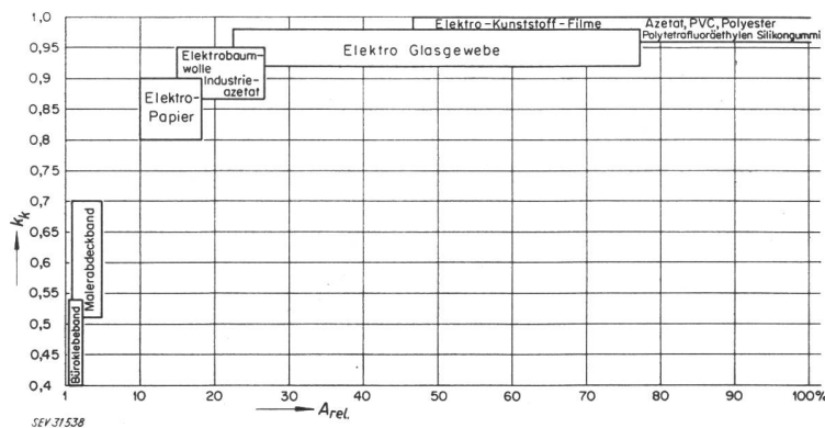
Fig. 8 Elektrolytischer Korrosionsfaktor und relative Alterungsbeständigkeit selbstklebender Elektroisolationen k_k elektrolytischer Korrosionsfaktor; A_{rel} relative Alterungsbeständigkeit
