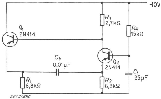
Fig. 1 Emitttergekoppelter Multivibrator
