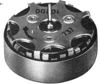
Offener Synchron-Langsamläufermotor SH 2
