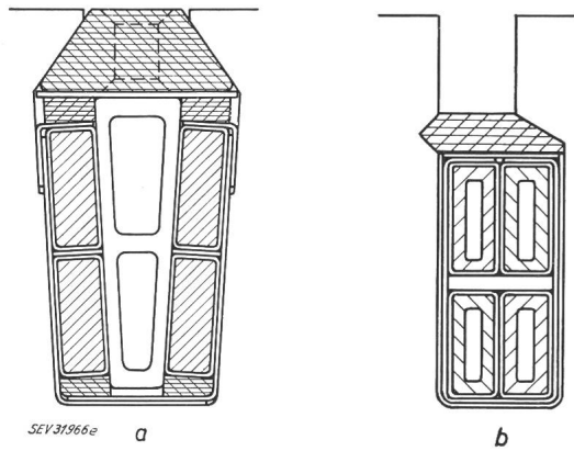
Fig. 15 Nutenschnitte eines Schleifringankers mit direkter Leiterkühlung a Kühlkanal in der Nutenmitte; b Hohlleiter
