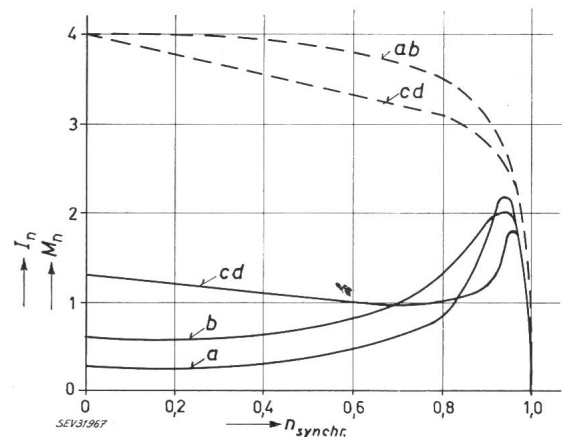
Fig. 16 Ausführungsarten von Rotorkäfigen und ihr Einfluss auf Strom- und Drehmoment-Verlauf bei Asynchronmotoren im Leistungsbereich 500...2000 kW
