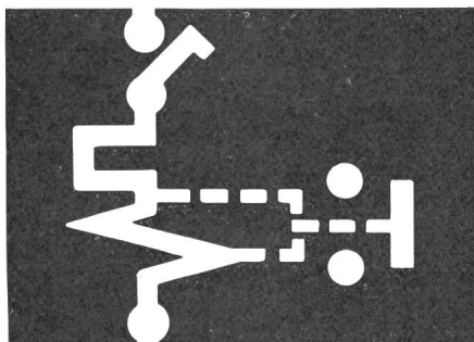
SL mit Signalkontakt
