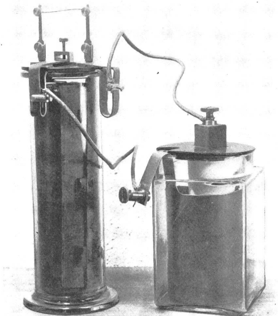
Fig. 11 Erste Anordnung zur Formierung der Blei-Elektroden eines Planté-Sekundärelementes
