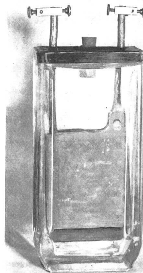
Fig. 12 Faure-Akkumulator Ausführung ca. 1910
