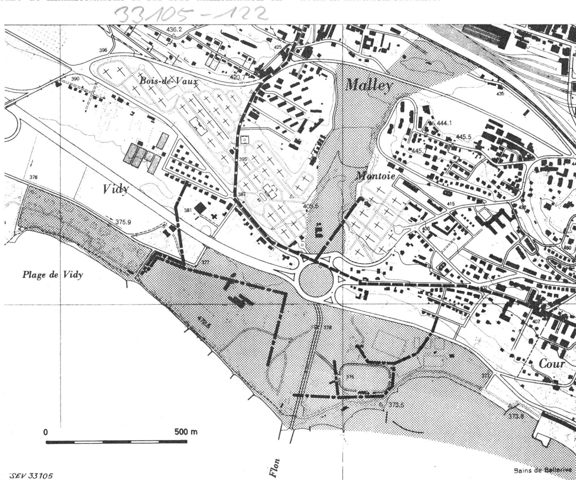
Fig. 1 Réseau 6 kV existant dans l'aire de l'Exposition Nationale au moment du choix de Vidy comme emplacement de cette manifestation
