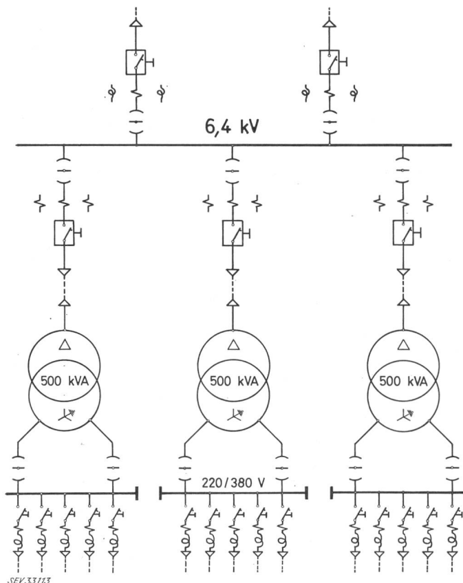
Fig. 9 Schéma de principe unipolaire des postes de transformation 6400/380 V
