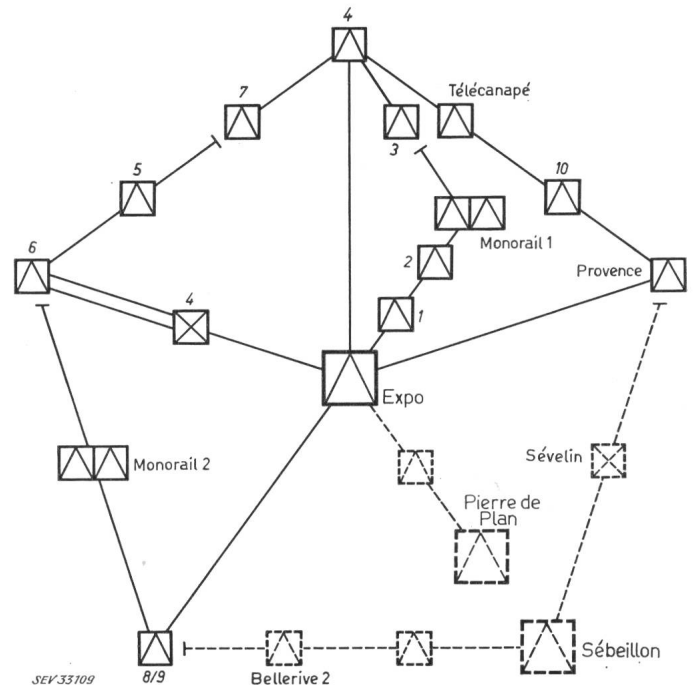
Fig. 5 Schéma de principe du réseau 6 kV de l'Exposition Nationale montrant les points de liaison avec le réseau moyenne tension lausannois — Exposition - - - S. E. L. ▽ Station de transformation ▣ Poste de couplage 1, 2, ... 10: N° des stations
