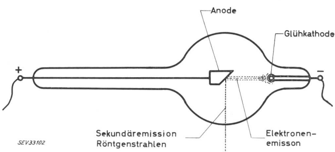
Fig. 9 Prinzipschema einer Röntgenröhre
