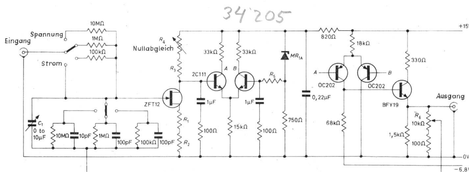
Schema eines Gleichstromverstärkers mit einem Feldeffekt-Transistor als Vorstufe Erklärungen siehe im Text
