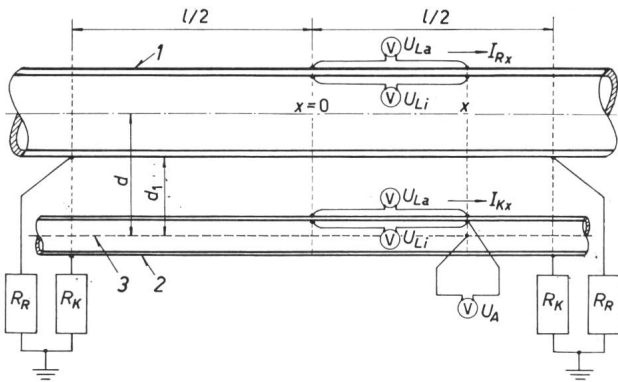
Fig. 3 Längsspannungen und Aderspannung 1 Rohrleitung; 2 Kabelmantel; 3 Kabeladern Weitere Bezeichnungen siehe im Text
