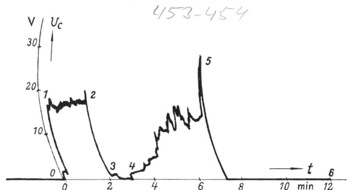
Fig. 1 Aufzeichnung von Teilentladungen U_c in einem Versuchsmuster aus Papier-Isolation, die unter einer Wechselfspannung von 10 kV mit Mineralöl getränkt wird
