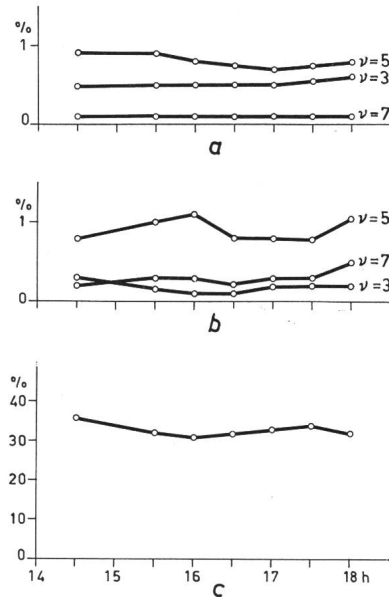
Fig. 3 Messwerte der Meßstelle Nr. 2 in Mettlen Leitung: Mettlen - Rathausen, 150 kV/100 MW Datum der Messungen: 13. April 1966 Bezeichnungen siehe Fig. 2 und Tab. I
