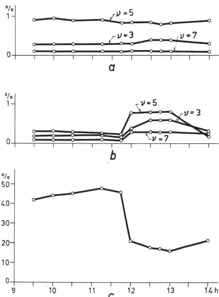
Fig. 2 Messwerte der Meßstelle Nr. 1 in Mettlen Leitung: Lavorgo - Gotthard - Mettlen, 220 kV/200 MW a Oberwellengehalt der Netzspannung; b Oberwellengehalt des Netzstromes; c relative Belastung der Leitung P/P_{max} \nu Ordnungszahl der Oberwellen Datum der Messungen: 13. April 1966
