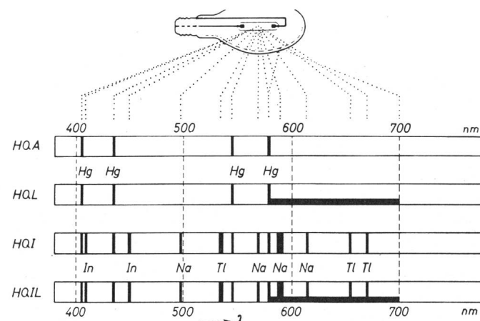
Fig. 5 Quecksilber-Hochdrucklampen Spektrale Bauart
