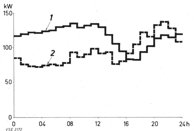
Fig. 2 Belastungsverlauf in Skellefteå an einem sonnigen Märztag 1 = 32 Häuser mit elektrischer Raumheizung 2 = 115 Häuser ohne elektrische Heizung
