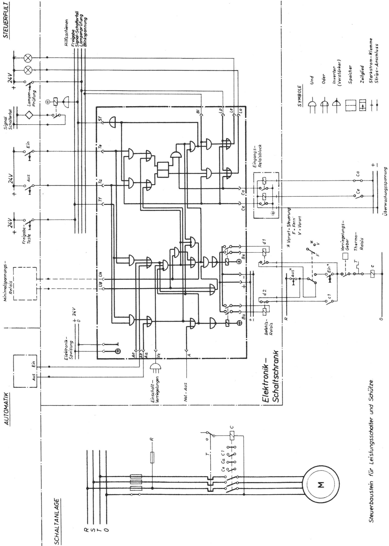
Fig. 3 Steuerbaustein für Leistungsschalter und Schütze Das Schaltbild zeigt die interne Logik und die äusseren Verbindungen des Stueurelementes, einerseits zum Steuerpult und dem Automatik-Steuergeraet und andererseits zur Schaltanlage. Dargestellt ist die Steuerung eines Motorschuetzes
