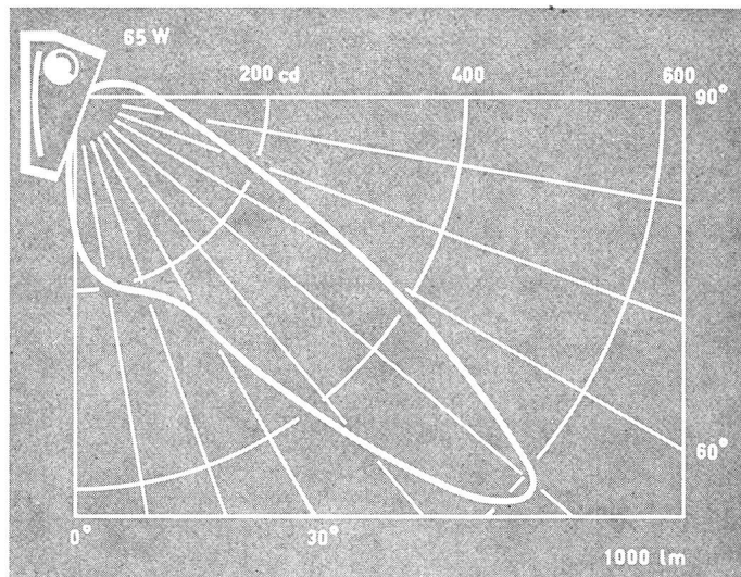
Fig. 1 Lichtverteilungsdiagramm der Reflektorleuchte Die Öffnung der Reflexschicht ist dem Reflektor zugekehrt
