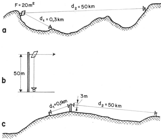
Fig. 8 Passive Reflektoren
