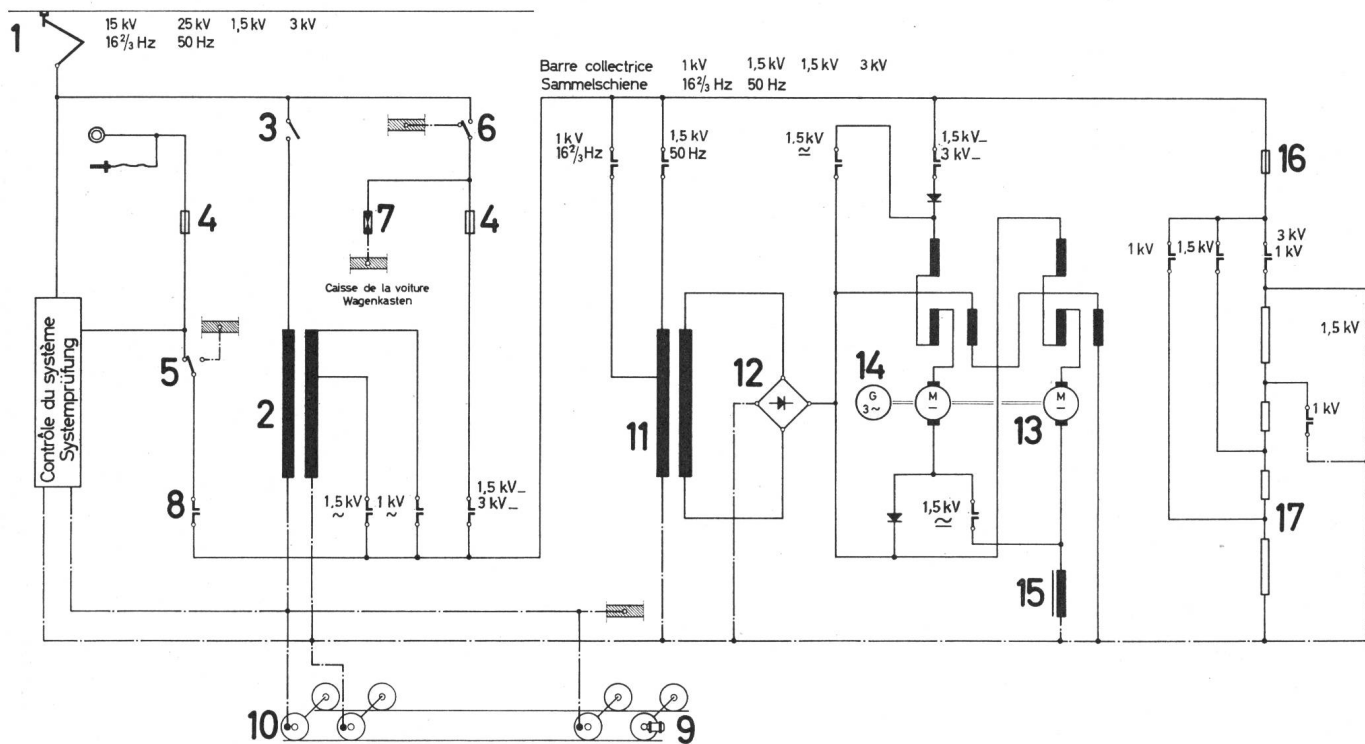
Fig. 4 Hauptstromkreise
