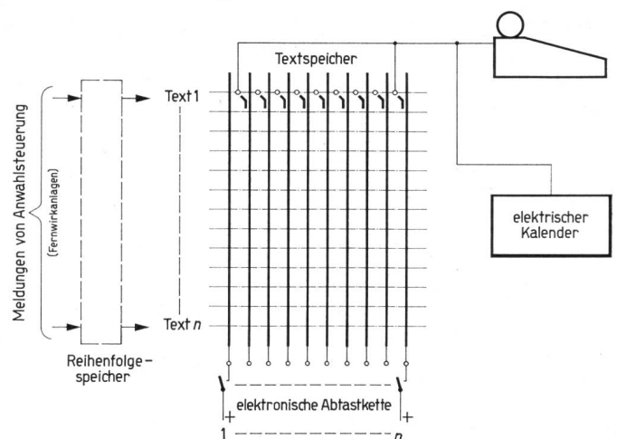
Fig. 8 Prinzipschema eines Informationsspeichers für die selbsttätige Protokollierung
