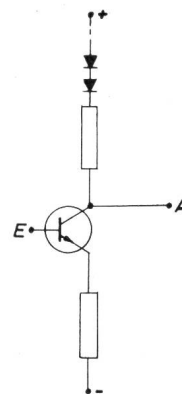
Fig. 1 Transistorstufe mit stabilerter Spannungsverstärkung E Eingang; A Ausgang
