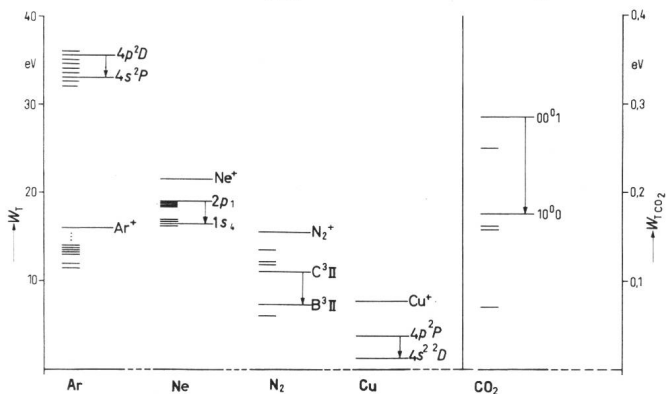
Fig. 4 Energetische Lage der Laserniveaus von Ar + , Ne, N 2 , Cu und CO 2 Die Ordinate bei CO 2 ist 100fach überhöht
