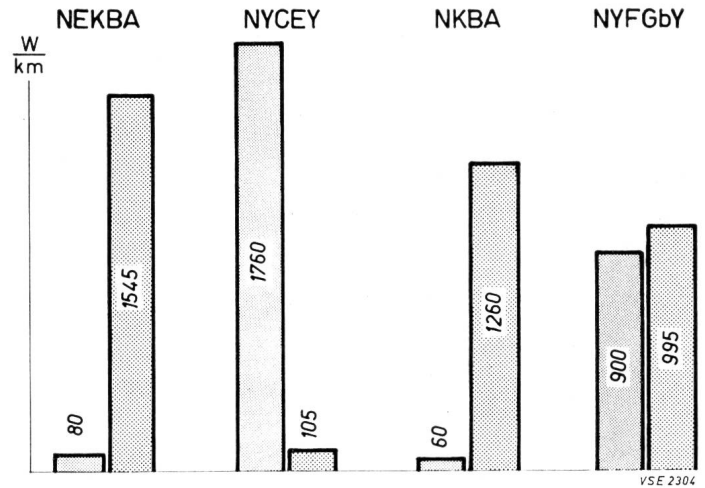
Fig. 15 Verluste und Zusatzverluste (nach Wehn) Parameter NEKBA NYCEY NKBA NYFGbY C_B ( \frac{\mu F}{km} ) 0,6 0,8 0,45 0,55 tg\delta 0,004 0,07 0,04 0,05 R_{zus} ( \frac{\Omega}{km} ) 0,012 0,001 0,0012 0,0095
