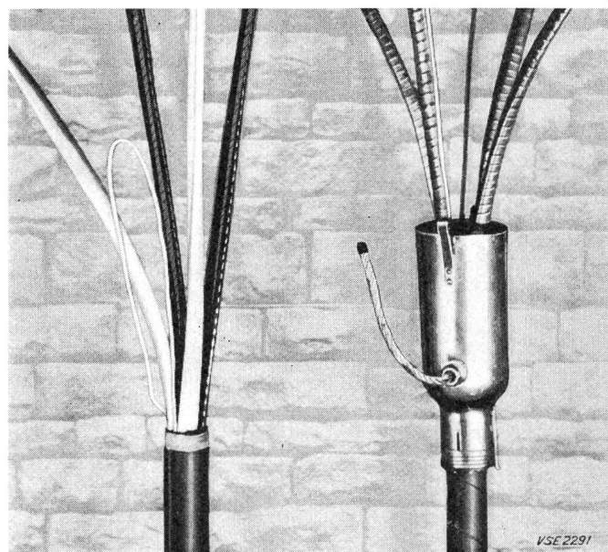
Fig. 2 Endabschluss Niederspannungs-Kunststoff- und Papierbleikabel
