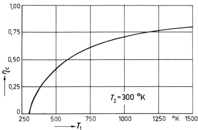
Fig. 3 Wirkungsgrad des Carnot-Kreisprozesses
