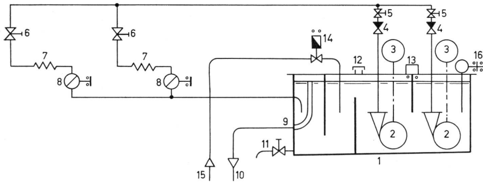
Fig. 11 Schema des Stehlagers-Kühlsystems
