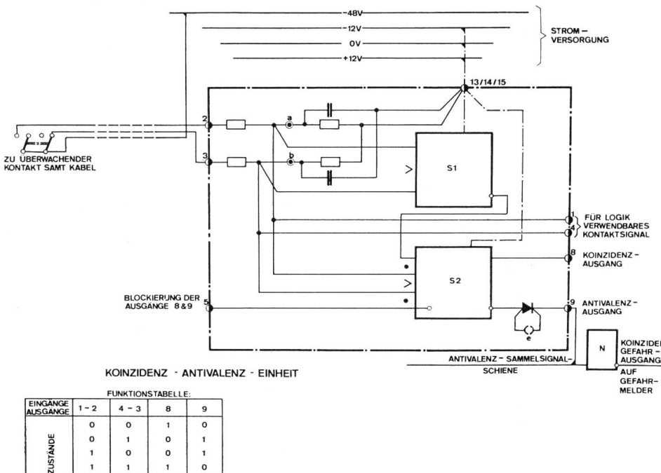
Schaltung einer Koinzidenz-Antivalenz-Einheit für die Geberkontakt- und Leistungsüberwachung
