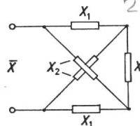
Fig. 1 Mit Reaktanz X abgeschlossene Zweigbrücke
