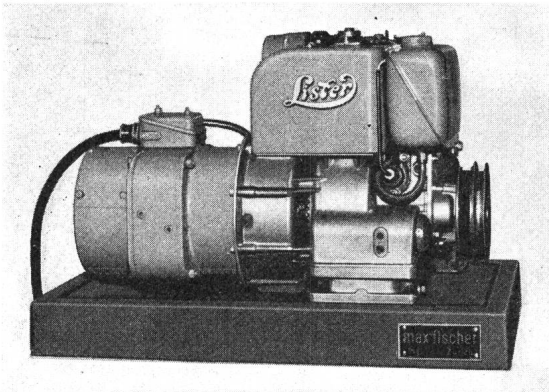
Fig. 1 Notstromgruppe
