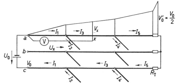
Fig. 3 Prinzip der Potentialabtastung
