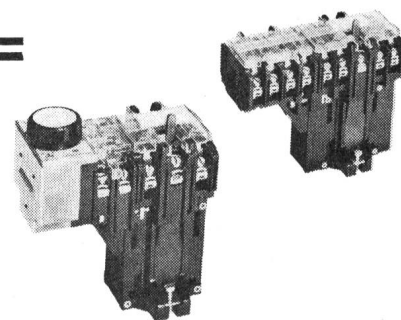
Hilfsblock mit 2 Kontakten zum nachträglichen Erweitern einer fertigen Steuerung, ohne deren Fläche zu vergrössern
