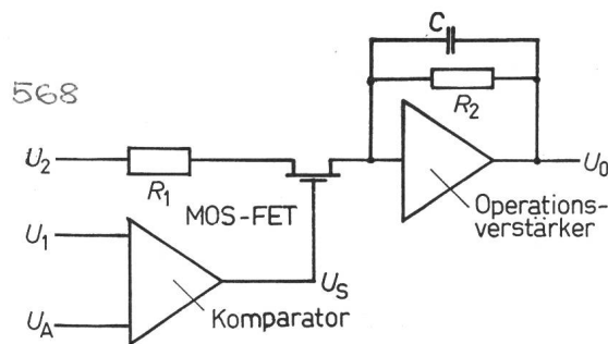
Fig. 1 Schematischer Aufbau eines Blockes Bezeichnungen siehe im Text
