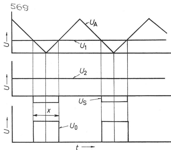
Fig. 2 Prinzip der Multiplikation Bezeichnungen siehe im Text
