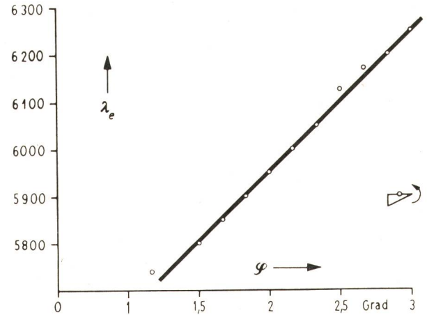
Fig. 15 Die Emission des Farbstofflasers als Funktion des Drehwinkels vom Prisma
