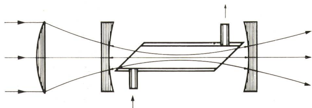
Fig. 12 Experimentelle Anordnung des FarbstoffLasers für longitudinales Pumpen, Brewster Küvette und Anpassungslinse für die Kaustik des konfokalen Resonators
