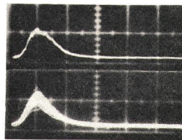
Fig. 11 Einzelimpuls und Schwankung der grünen Emission (10 ns)
