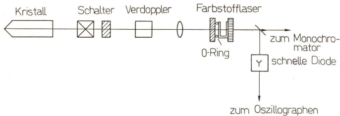
Fig. 9 Schematische Darstellung des RiesenimpulsLasers mit Frequenzumsetzung
