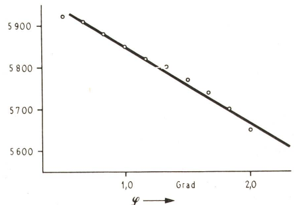
Fig. 16 Die Emission des Farbstofflasers als Funktion des Drehwinkels vom Gitter
