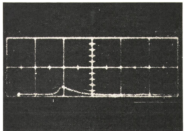
Fig. 20 Farbstoffimpuls von 2 ns Dauer Der Resonator ist 5 mm lang (2 ns/Div)
