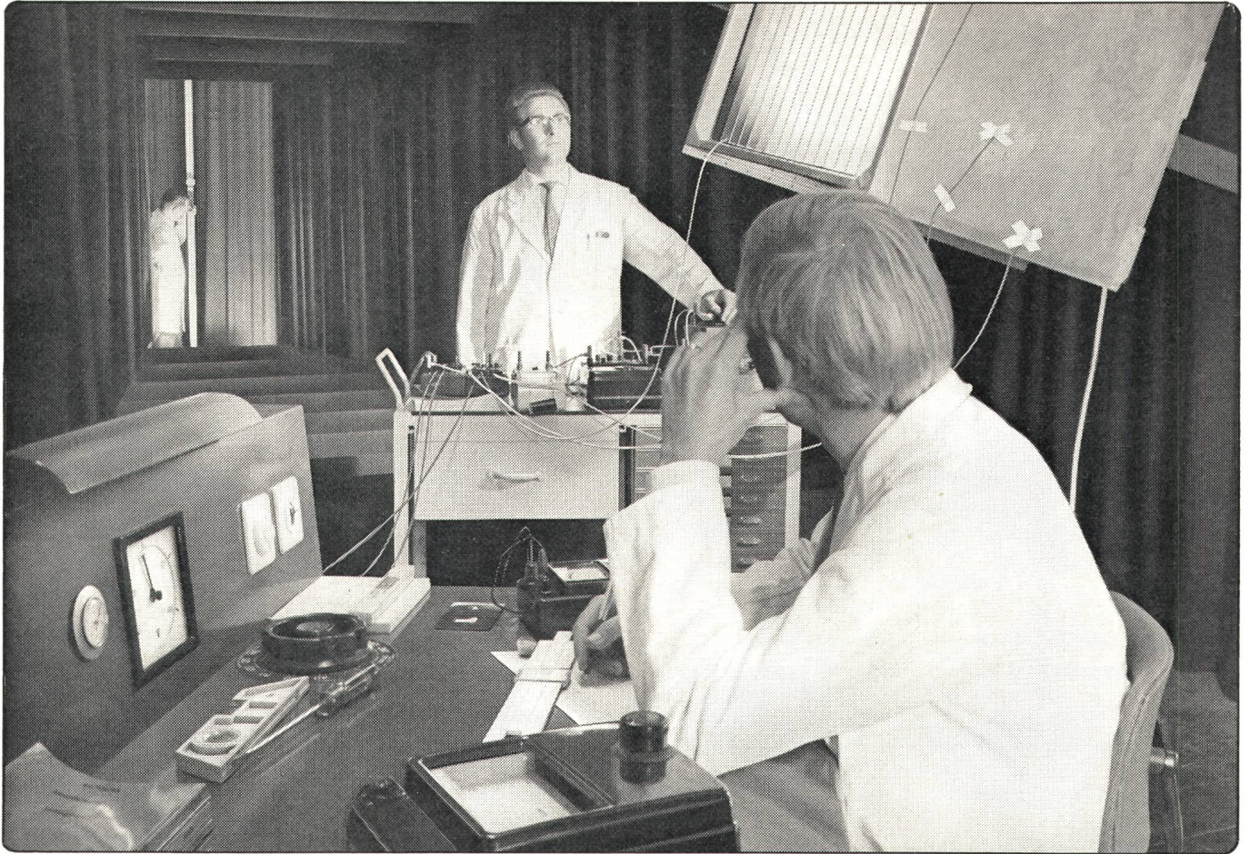
Messungen zum Problem der Beleuchtung von Tunnelleinfahrten im lichttechnischen Labor der Zürcher Firma Alumag-Belmag AG.
