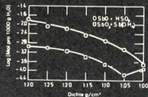
Fig. 14 Löslichkeitskurven und Antimonien in Schwefelsäure nach Rutschki und Angstadt (1)
