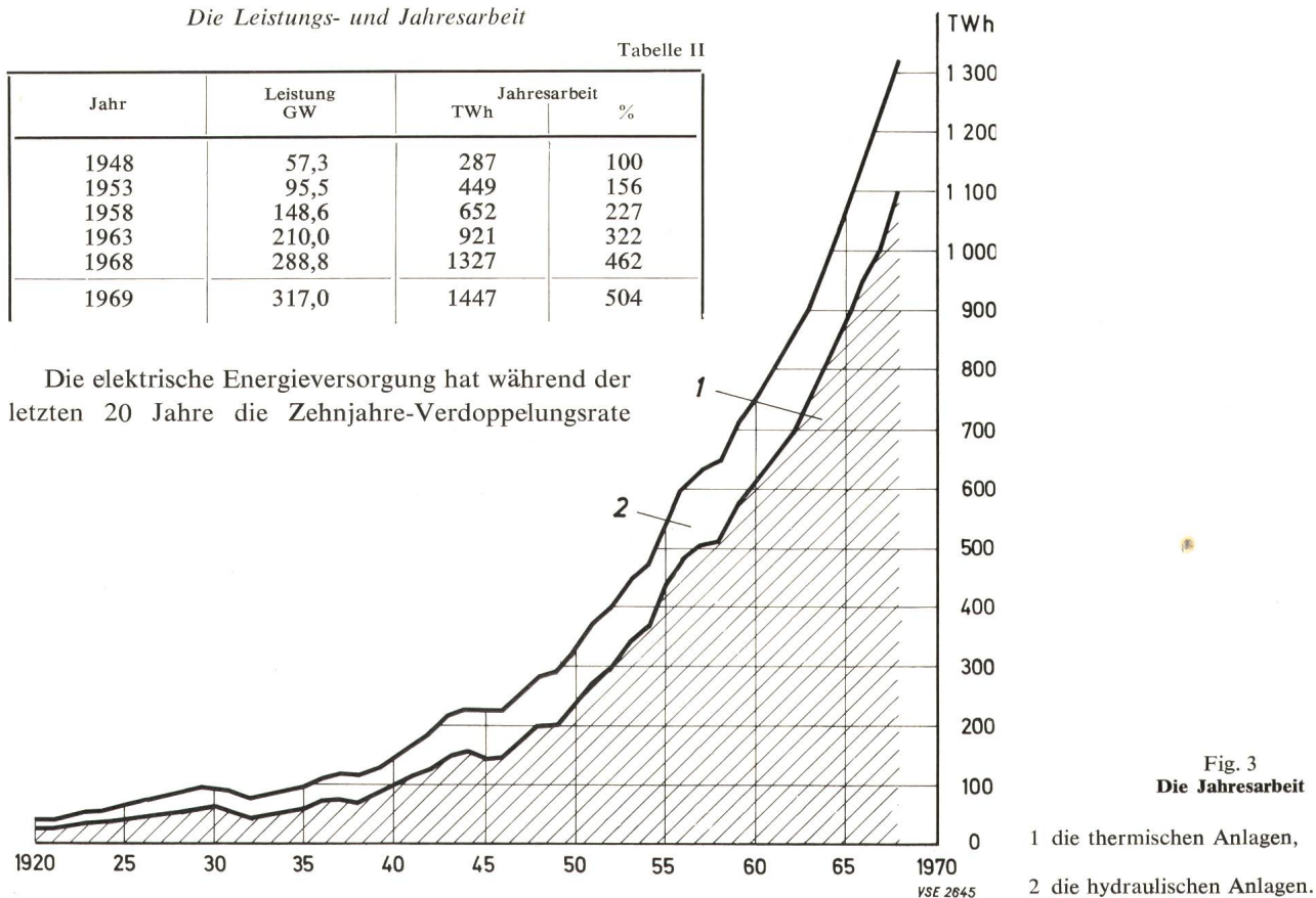
Die Leistungs- und Jahresarbeit
