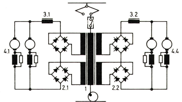
Fig. 1 Principalschema der Hauptstromkreise für Fahrbetrieb 1 Transformator; 2 Stromrichter; 3 Glättungsinduktivitäten; 4 Triebmotoren
