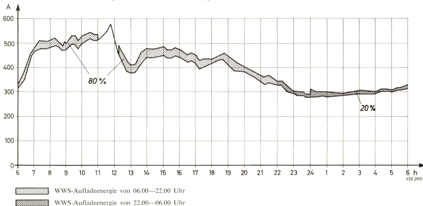
Diagramm 1b Belastung einer 13-kV-Unterstation (Sperrzeit für WWS von 11.00 bis 12.15 Uhr)
