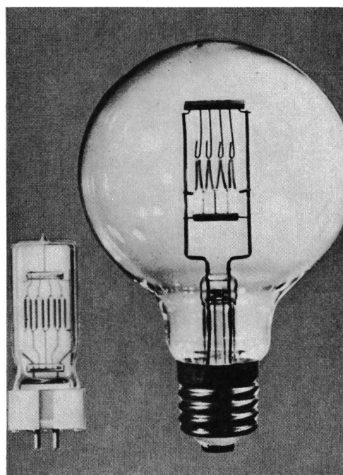
Fig. 6 Grössenvergleich: Lampe 1000 W für Fernseh- und Filmstudio-Halogenlampe zu konventioneller Glühlampe
