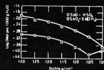
Fig. 14 Löslichkeitskurven und Antimonionen in Schwefelsäure nach Ruetschi und Angstadt (7)
