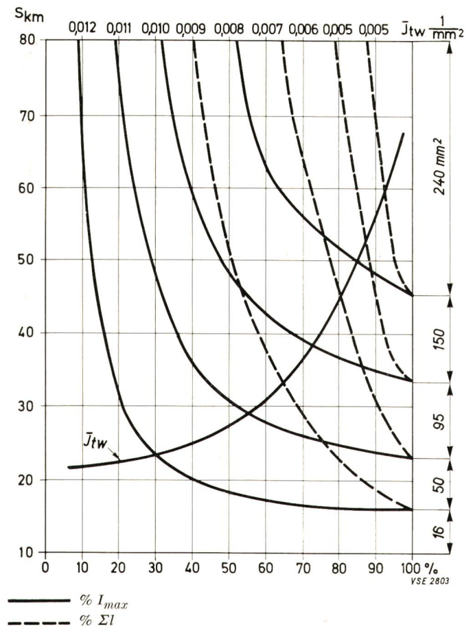
Fig. 1 Auswahl der Leiter aus einem Querschnittssortiment von 16 — 50 — 95 — 150 — 240 mm 2 % I max Stromgrenzen der Querschnitte % Σl Anteil der Querschnitte an der totalen Leitungslänge \bar{j}_{tw} Relative Stromdichte der Leitungen \hat{s}_{km} Mittlerer kommerzieller Querschnitt
