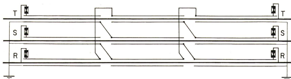
Fig. 1 Kabelanlage mit ausgekreuzten Mänteln und mit Überspannungsableitern zwischen Leitern und Erde Prinzipisches Schema
