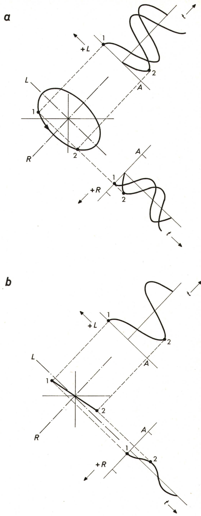
Fig. 22 Abtastbewegung des Diamanten bei gegebenem Beispiel a bei einer quadrophon bespielten Platte b bei einer stereophon bespielten Platte Weitere Bezeichnungen siehe Fig. 1 und 18
