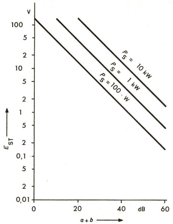
Fig. 5 Stör-EMK E_{ST} am Empfänger-Eingang für R_i = 50 \Omega
