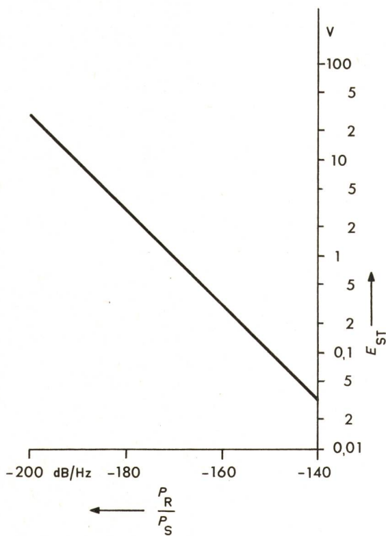
Fig. 6 Zusammenhang zwischen zulässiger Stör-EMK E_{ST} und Senderrauschabstand P_R/P_S
