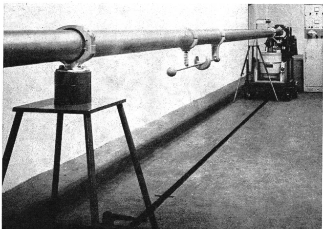
Fig. 8 Rohrschwingungsstand
