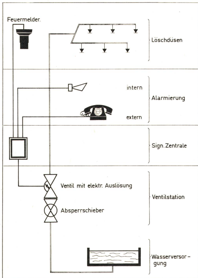
Fig. 12 Prinzip einer Sprühflutanlage
