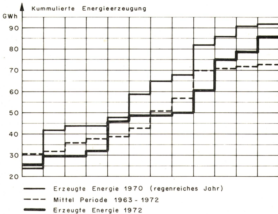
Fig. 12 Monatliche Energieerzeugung der eigenen hydraulischen Kraftwerke der BKW.
