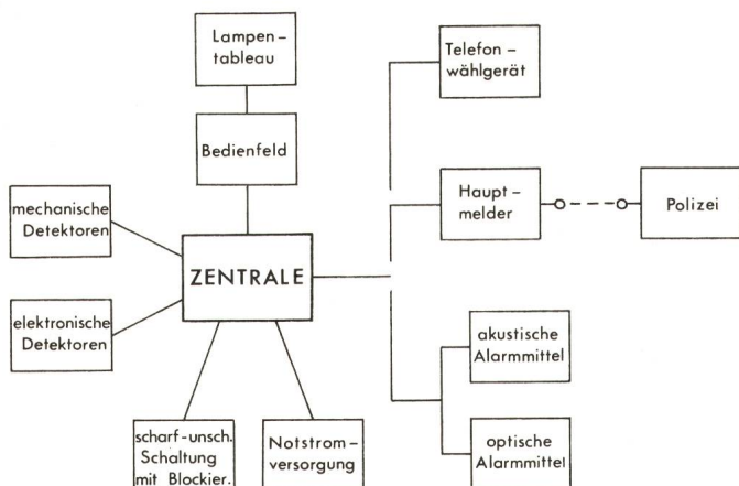
Fig. 1 Blockschaubild einer elektrischen Sicherungsanlage
