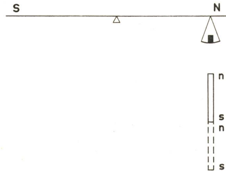
Fig. 6 Magnetische Waage Messung des Hauptflusses n, N Nordpole s, S Südpole
